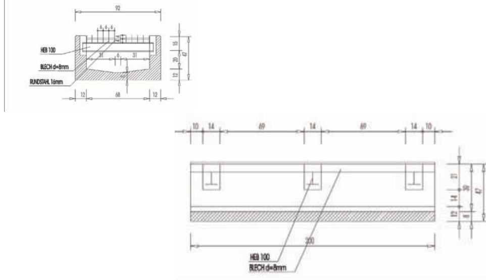
Abb. 7: Prinzipskizze und Maße eines Gitterrostes (SKIZZE: Büro FELBER-RICHTER, Salzburg)
